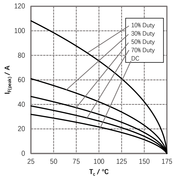
图 4. 电流降额
