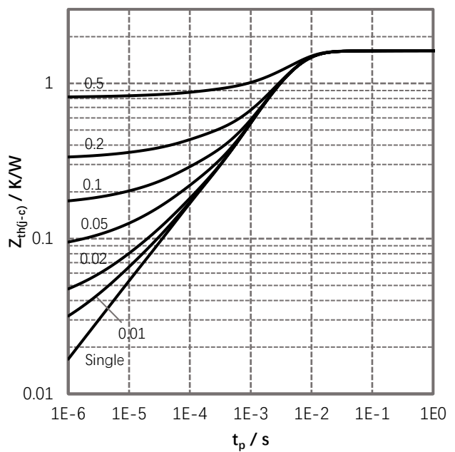
图 8. 瞬态热阻抗
