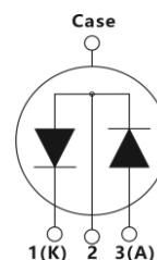
内部电路
