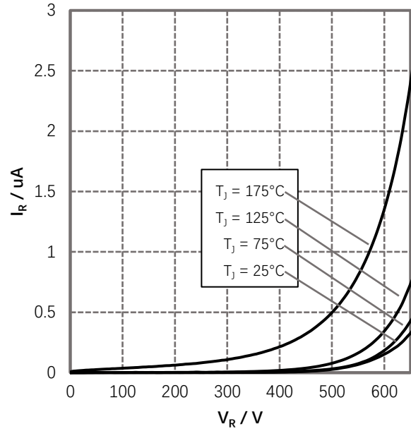
图 2. 反向特性
