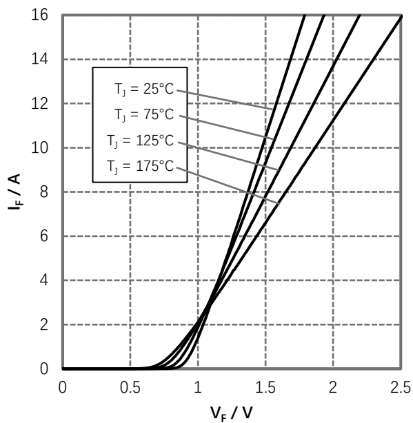
图 1. 正向特性
