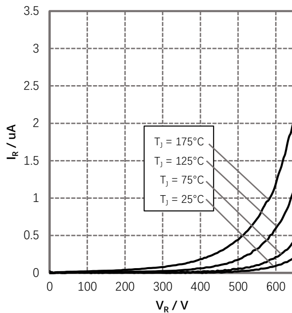
图 2. 反向特性
