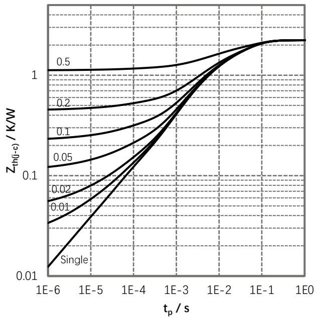
图 8. 瞬态热阻抗
