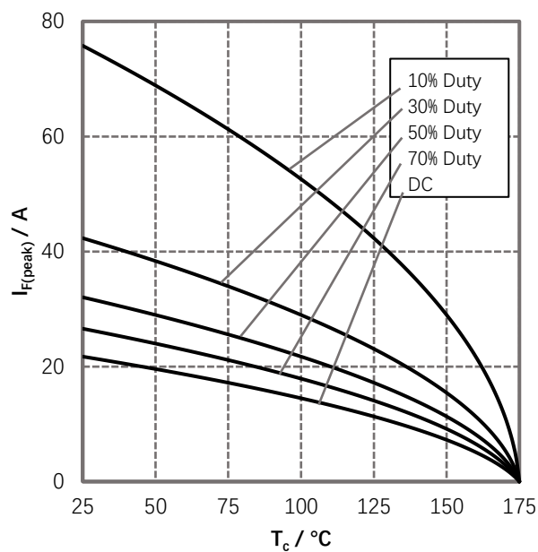
图 4. 电流降额
