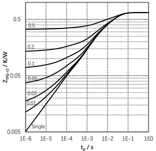
图 8. 瞬态热阻抗
